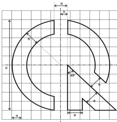
Hình 3. Kích thước cơ bản của dấu hợp quy
